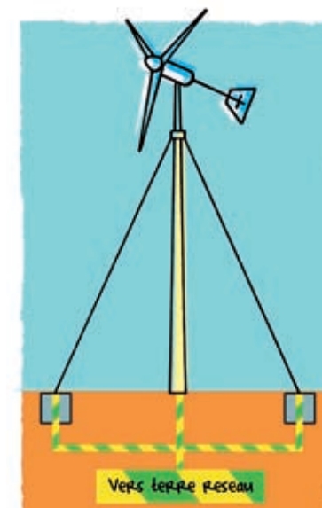
LA MISE À LA TERRE SE FAIT PAR DES FILS DE CUIVRE NUS DE 12,5 MM, INTERCONNECTÉS ENTRE EUX ET RELIÉS À LA MISE À LA TERRE DU RÉSEAU DOMESTIQUE. SIGNALONS QUE DANS LE CAS D'UN MÂT HAUBANÉ, LE FIL DE CUIVRE DOIT ÊTRE RACCORDÉ SUR LES HAUBANS AFIN QUE LA FOUDRE NE PASSE PAS PAR LES SOCLES EN BÉTON.
